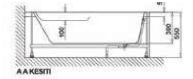
AA KESİTİ
