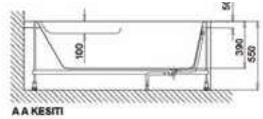
AA KESİTİ
