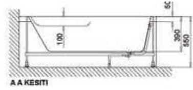
AA KESİTİ
