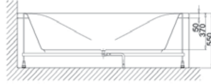
A A KESİTİ
