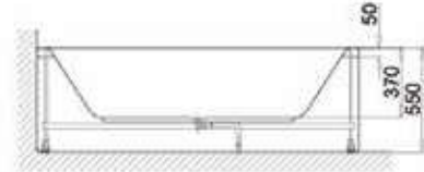
A A KESİTİ
