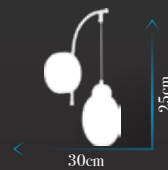
Kod | PV 123-1 CH APLİK Led Max. 2,5W / 6000 K Ölçü | W : 30cm H : 25cm
