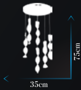
Kod | AD-101-5+1 FGD Led Max. 17W / 4000 K Ölçü | W : 35cm H : 75cm
