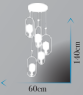
Kod | MTT023-5'Lİ Duy | E14 Max. 5 x 28W Ölçü | W : 60cm H : 140cm
