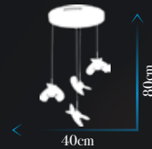
Kod | AD-086-4 FGD Led Max. 19W / 4000 K Ölçü | W : 40cm H : 80cm
